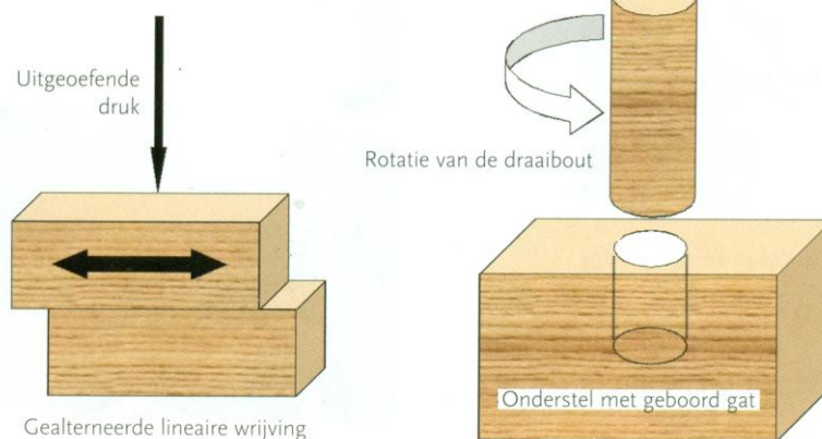
Figuur 1. De twee lasmethodes door wrijving
