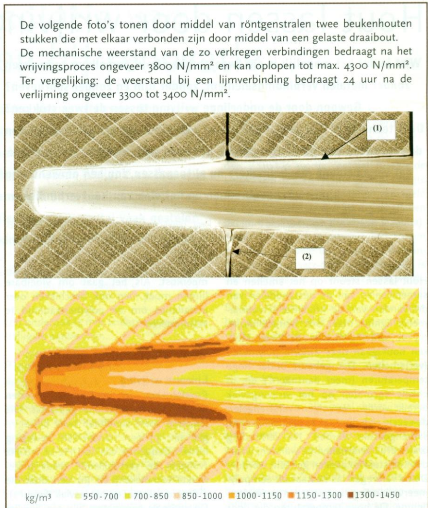
Figuur 2. Cirkelvormige wrijving
